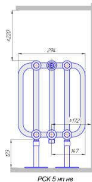
Радиаторы "РСК нп нв", монтажные схемы
